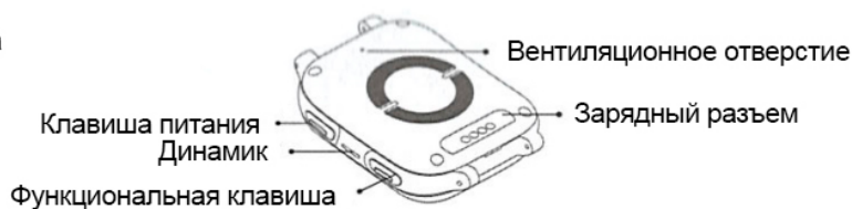
Задняя панель:
